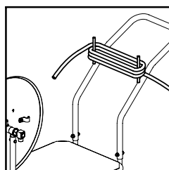
Supporto tubo di alimentazione Hose rest
